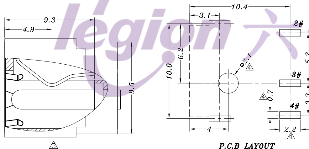
P.C.B LAYOUT
